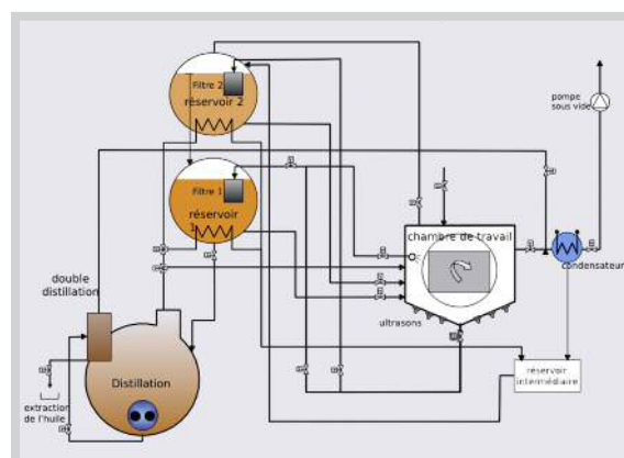
Schéma du déroulement du procédé sur RCTS „petite“
